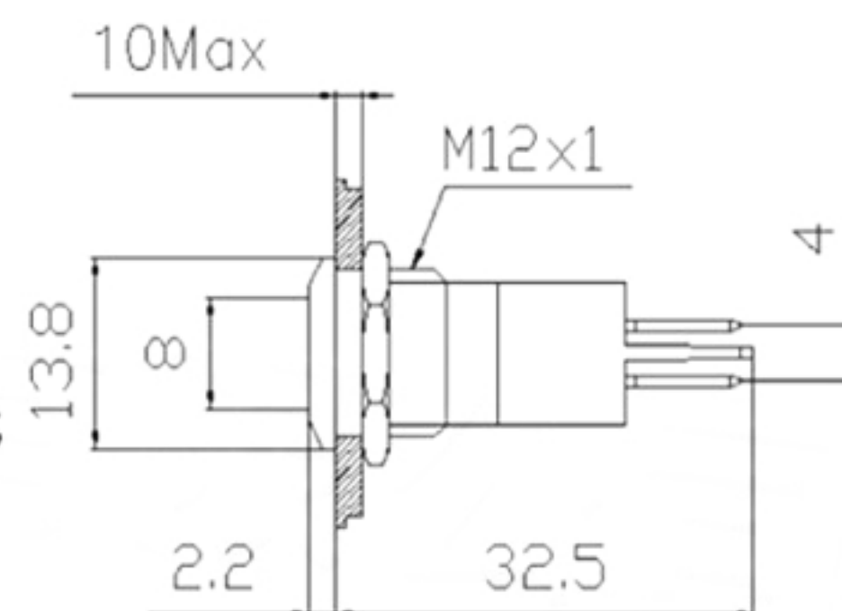
外形尺寸 Diameter
