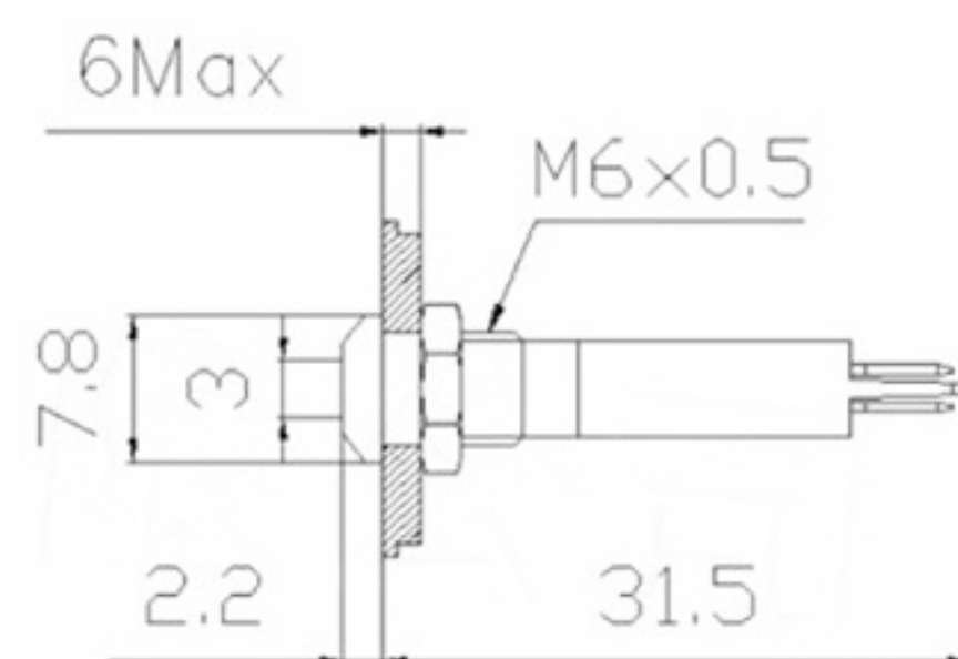
外形尺寸 Diameter
